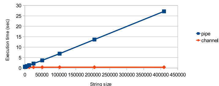
図 8 文字列と配列の転送速度
