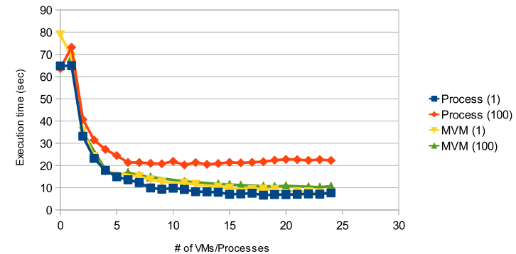
図 9 HTML 生成アプリケーションの結果
