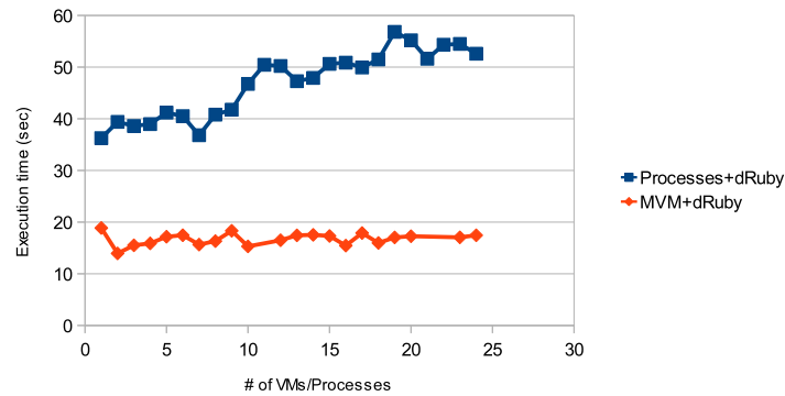
図 10 DB アプリケーションの結果
