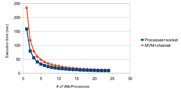
図 11 AO Bench の結果
